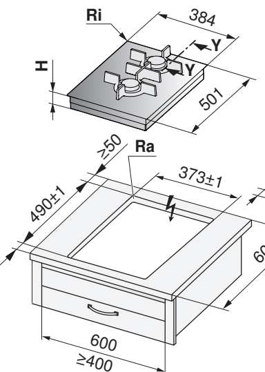
GAS421GSAZ/GSBZ (31064)
