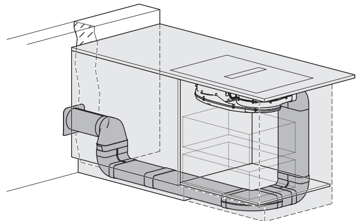
Uscita laterale dell'aria di scarico attraverso lo zoccolo
