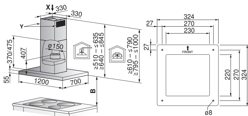
Schema di foratura (vista X)
